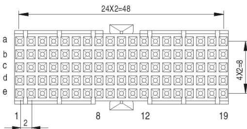
Type AB19(95 Pins)
