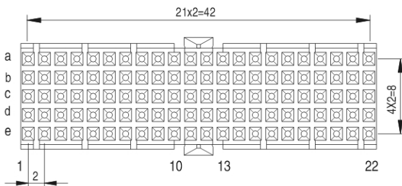
Type AB19(95 Pins)
