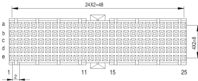
Type AB22(110 Pins)
